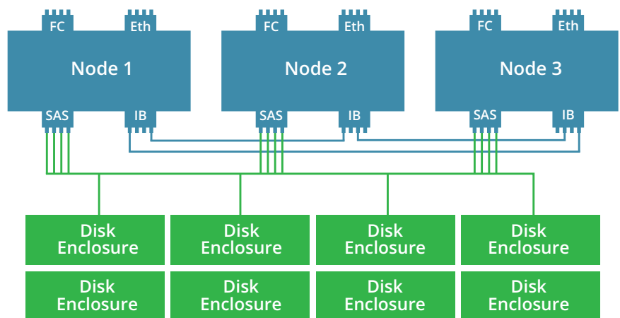
BILD 2 InfiniBox Frontend- und Backend-Konnektivität
